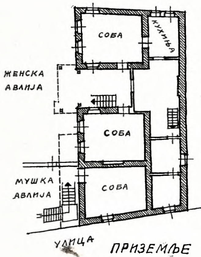
КУЋА „ФЕРИЗБЕГ АЛИЈЕ“
