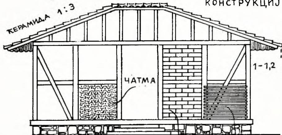
РАЗНИ НАЧИНИ ИСПУНЕ ЗИДОВА
