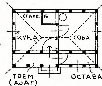
БАСКИЈЕ (КУЋА „КОВАНИЦА“)
