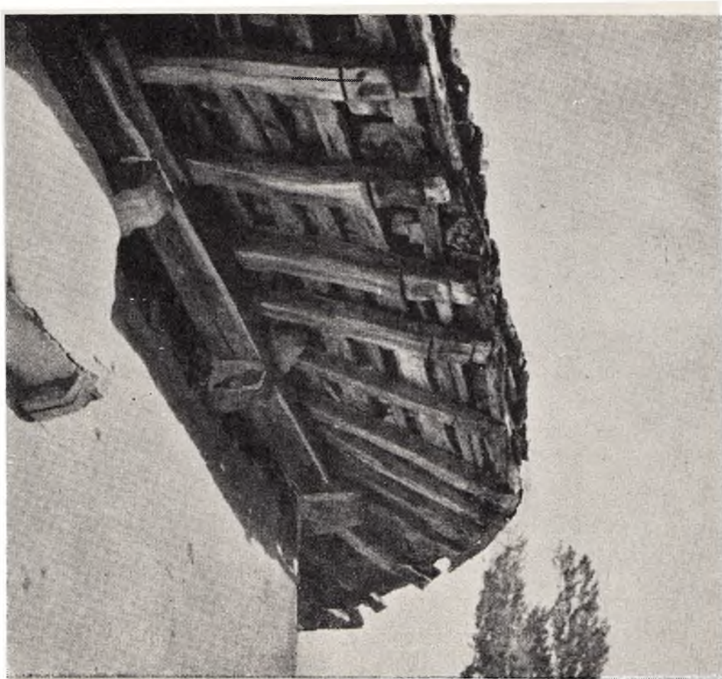
Сл. 20 — Стреја крова покривеног ћерамидом; рогови су оздо видни; олука нема
