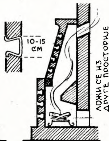
ПЕЋ СА "ЛОНЧИЋИМА"
