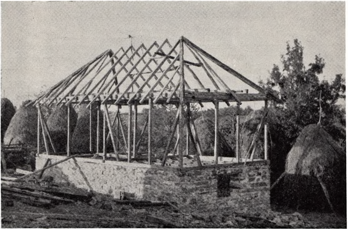
Сл. 14 — Сеоска кућа „бондручара” у грађењу. Подрум је озидан каменом а изнад њега се види скелет од гредица за зидове, који ће бити испуњени лакшим материјалом; кров је увек четворосливан (Србија)
