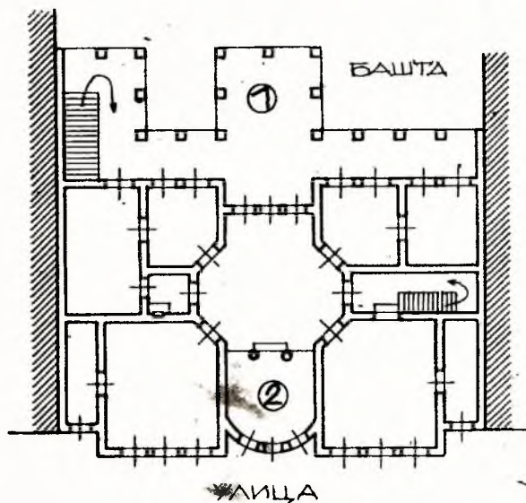
„ИЧКОВА КУЋА“ У БЕОГРАДУ ① ДОКСАТИ ② ДИВАНХАНЕ
